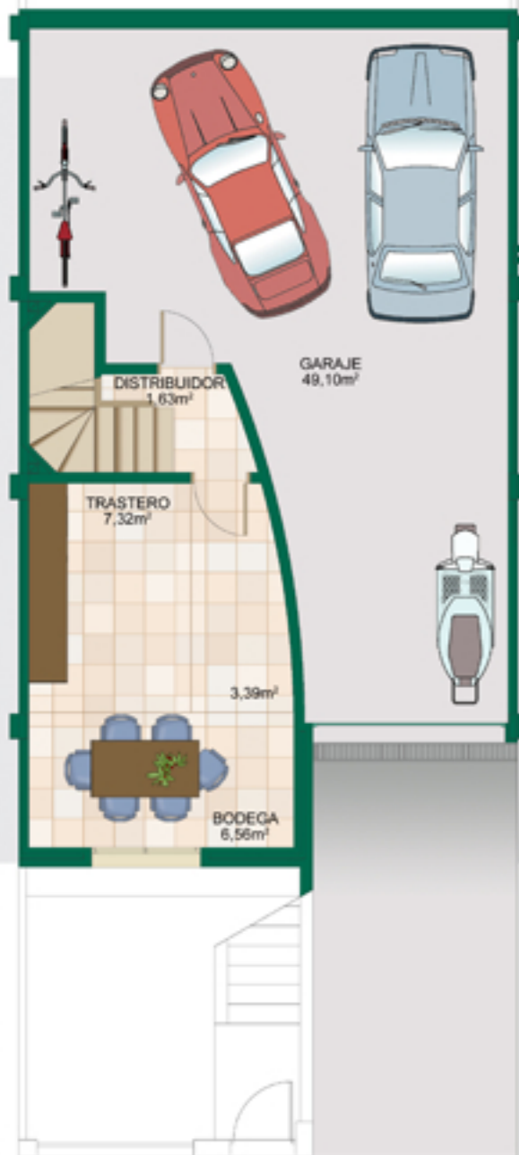
PLANTA SÓTANO
